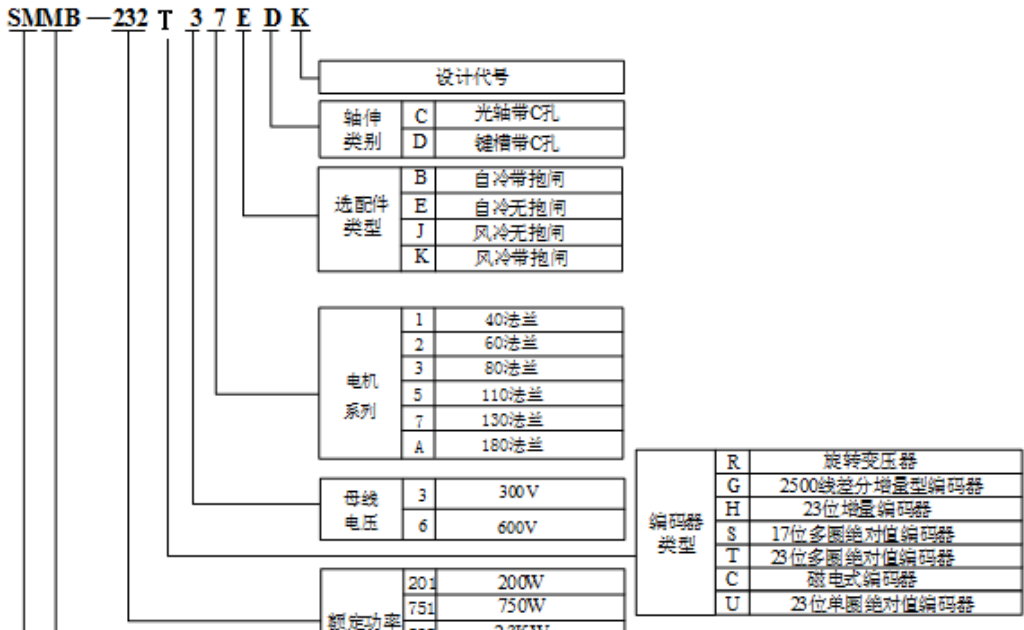
图 2.2.1 伺服电机命名规则（180 及以下法兰电机）
