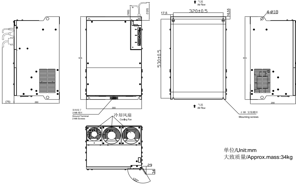
图 3.1.12 伺服驱动器结构尺寸 12
