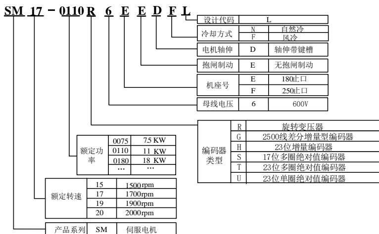
图 2.2.1 伺服电机命名规则（180 及以下法兰电机）
