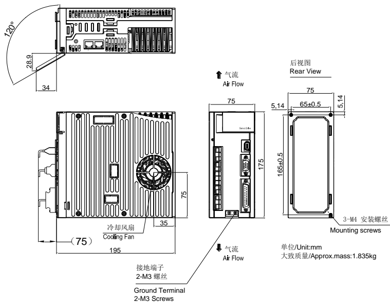
图 3.1.4 伺服驱动器结构尺寸 4
