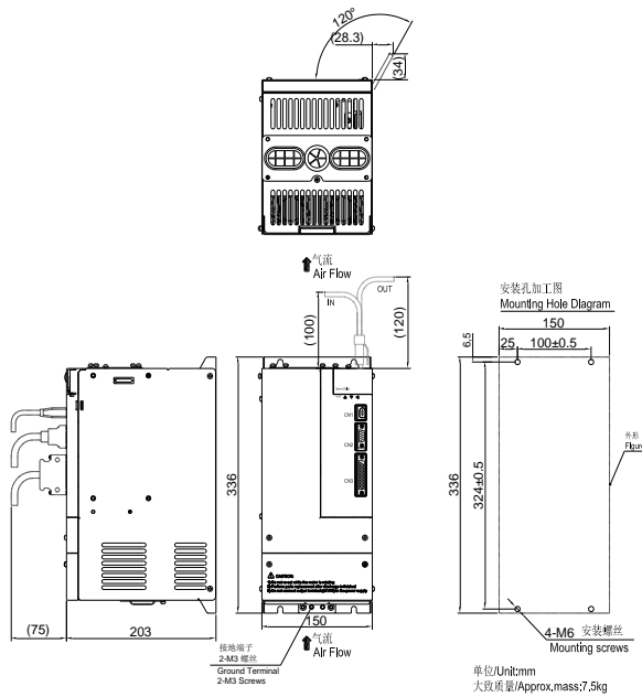
图 3.1.7 伺服驱动器结构尺寸 7
