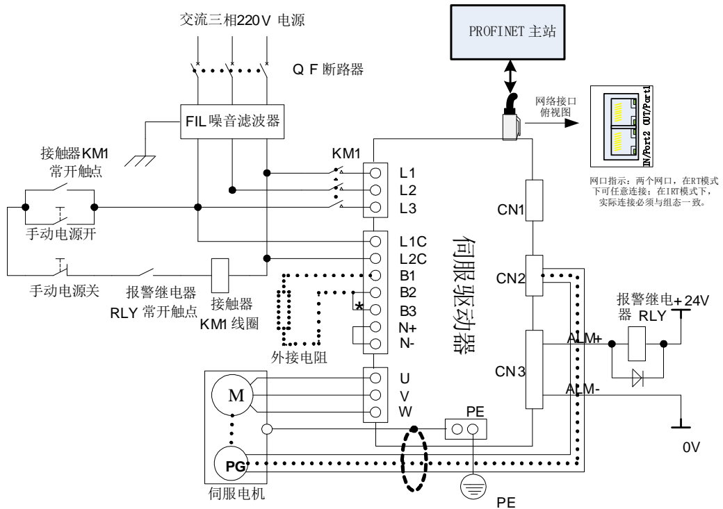
图 4.1.7 220V 驱动器典型主电路配线图
