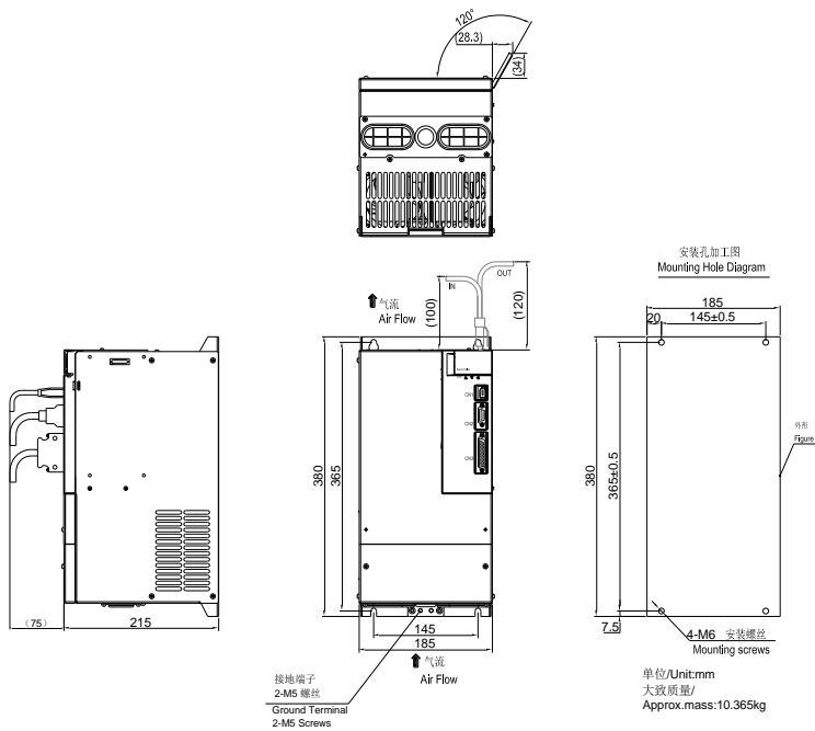
图 3.1.8 伺服驱动器结构尺寸 8
